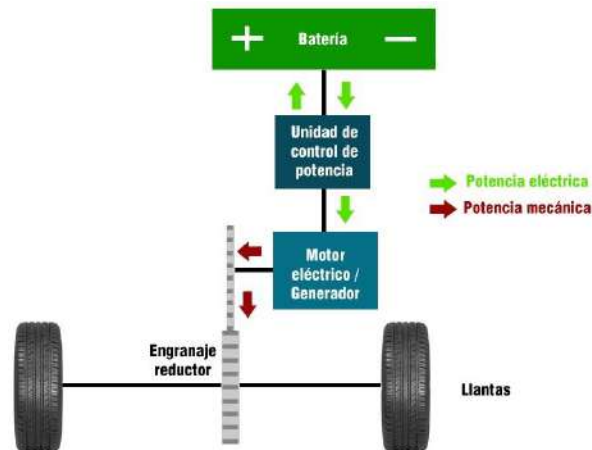
Figura 1.10 Esquema de un tren motriz de un vehículo híbrido en serie-paralelo
