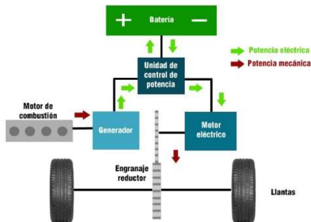
Figura 1.7 Esquema de un tren motriz de un vehículo híbrido en serie
