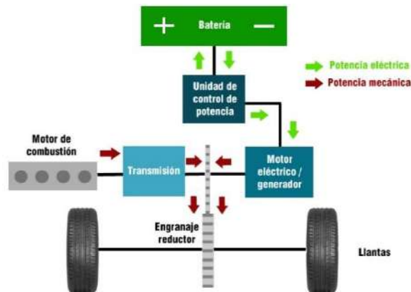
Figura 1.8 Esquema de un tren motriz de un vehículo híbrido en paralelo
