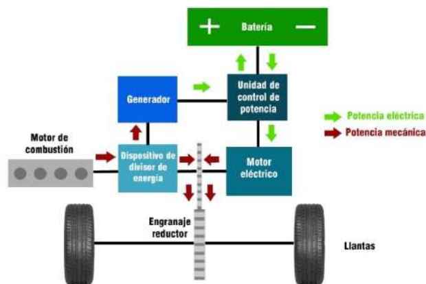
Figura 1.9 Esquema de un tren motriz de un vehículo híbrido en serie-paralelo
